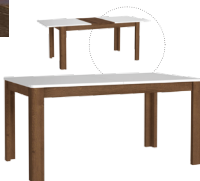
Stół rozkładany FLOT16 szer. 160 (207)/wys. 73/gł. 90 cm Dekor: L92
